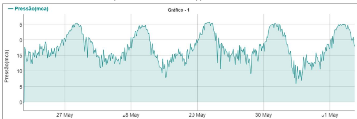
Figura 4 – Gráfico do data logger anexo à carta 654/2026
