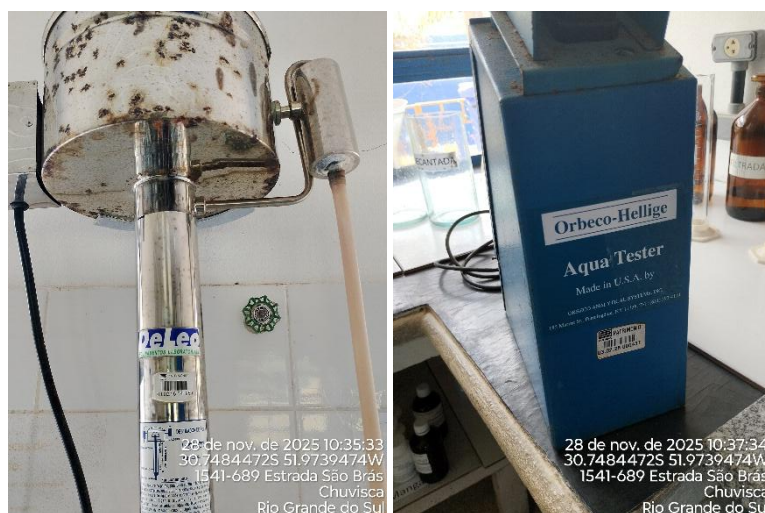
Figura 01: Equipamentos de laboratório existentes na ETA
