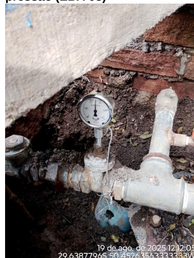
Figura 15: Transdutor de pressão (EBA 03)
