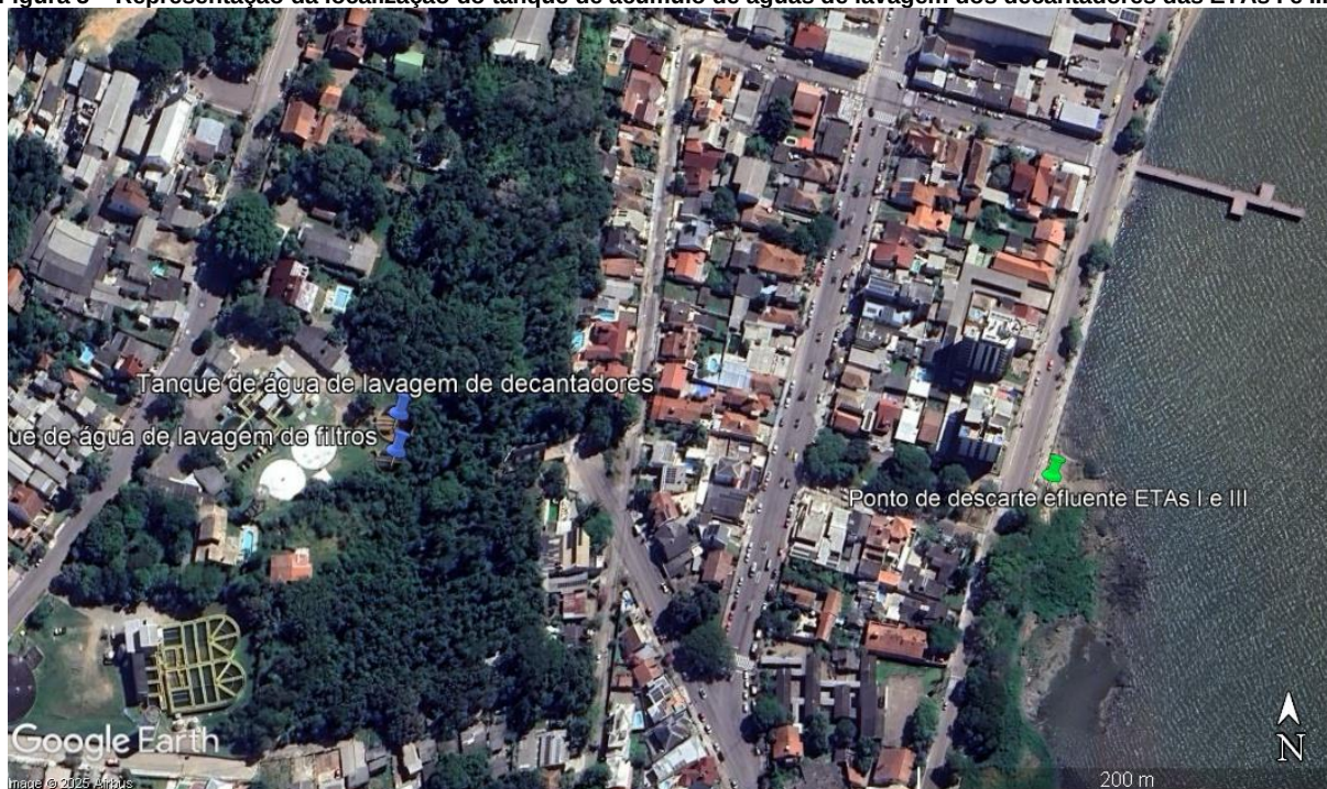
Figura 5 – Representação da localização do tanque de acúmulo de águas de lavagem dos decantadores das ETAs I e III.
