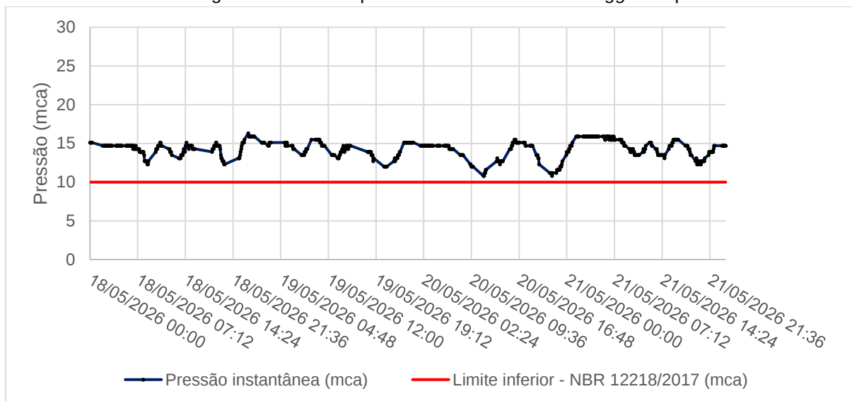
Figura 5 – Perfil de pressões obtido com Data Logger no ponto 3
