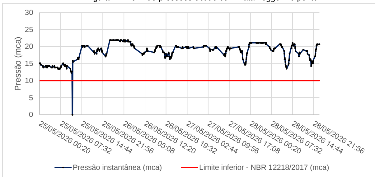
Figura 4 – Perfil de pressões obtido com Data Logger no ponto 2
