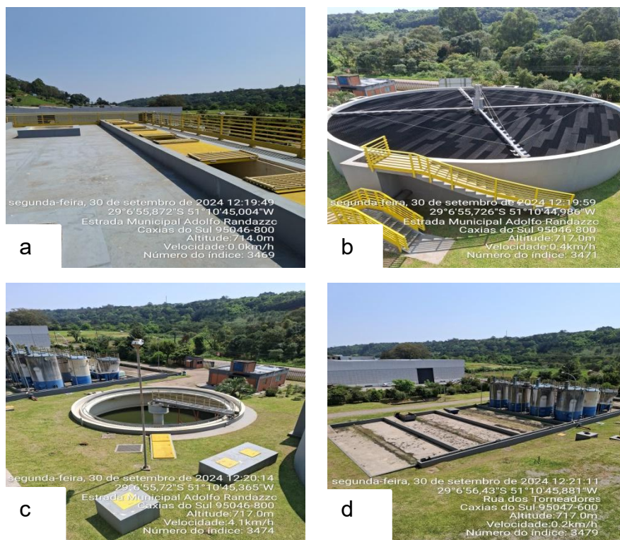
Figura 01: Obras em andamento na ETE Canyon de Caxias do Sul. a) Vista superior da etapa do reator; b) vista do filtro; c) vista do decantador; d) vista da ETE compacta em operação e leitos de secagem do lodo.
