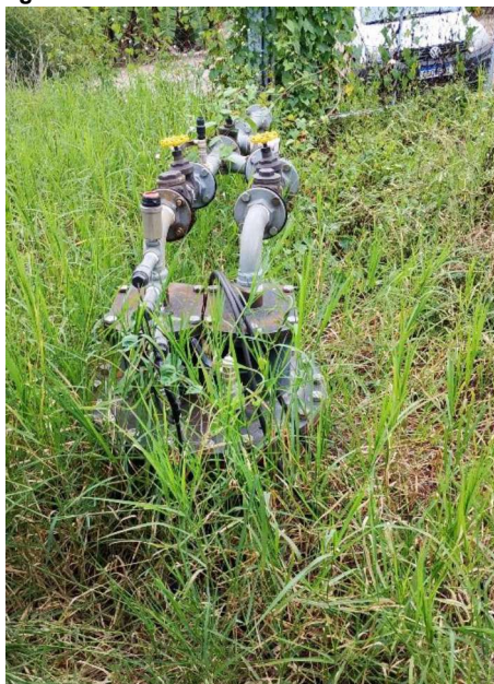
Figura 2 – EBAT associada ao reservatório 11.
