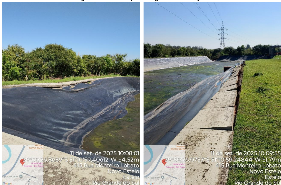
Figura 4 – Talude rompido na lagoa de estabilização.
