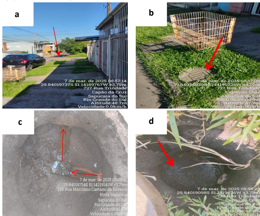
Figura 3 – Relatório fotográfico da fiscalização in loco . A) Identificação da área frontal do imóvel (destaque em vermelho indica o Poço de Visita (PV) existente nas proximidades; b) Identificação da caixa de ligação existente na calçada do imóvel; c) Vista interior do Poço de Visita (PV) localizado nas proximidades do endereço; d) Vista do interior da caixa de ligação do imóvel em questão.
