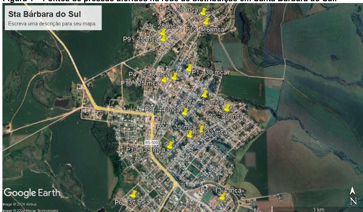
Figura 1 – Pontos de pressão aferidos na rede de distribuição em Santa Bárbara do Sul.
