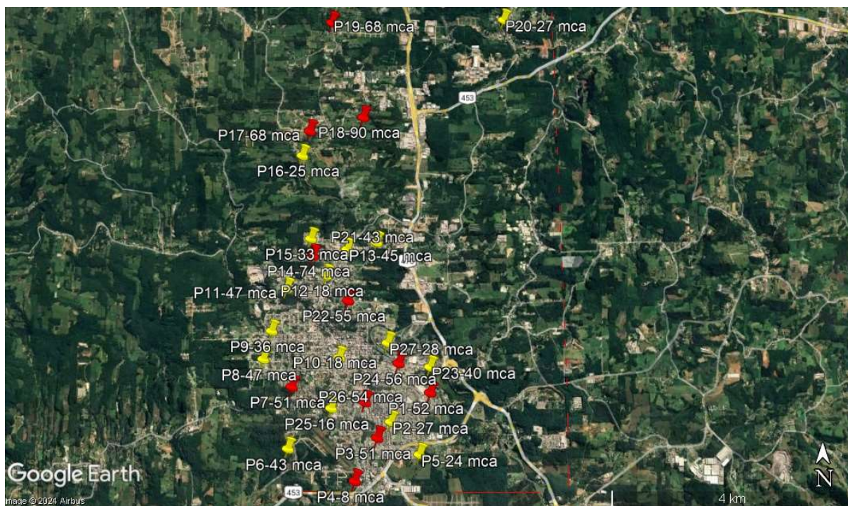
Figura 1 – Pontos de pressões aferidas na rede de distribuição em Garibaldi.
