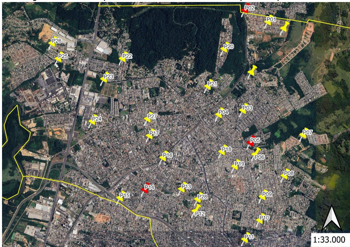
Figura 1 – Pontos de pressão aferidos na rede de distribuição em Sapucaia do Sul.
