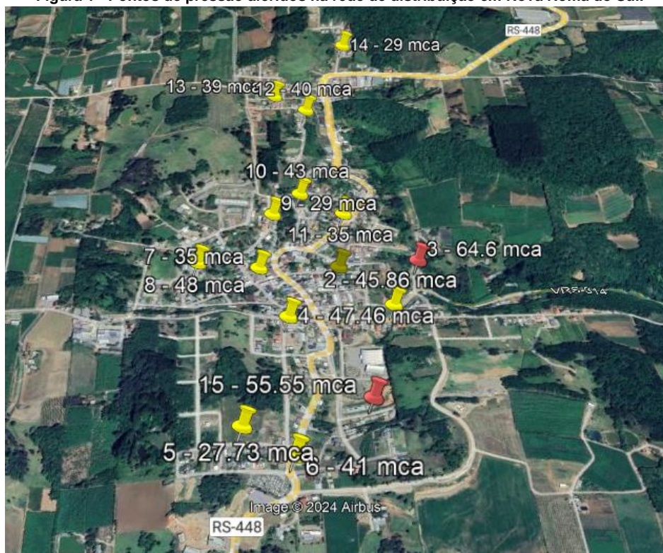
Figura 1 - Pontos de pressão aferidos na rede de distribuição em Nova Roma do Sul.
