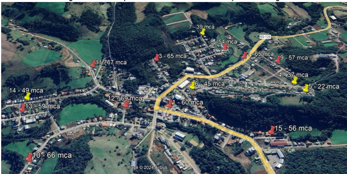
Figura 1 - Pontos de pressão aferidos na rede de distribuição em São Jorge.
