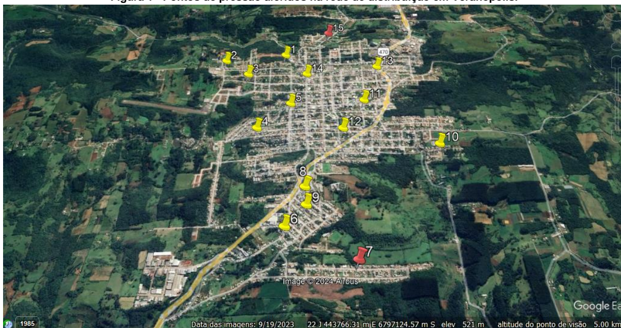
Figura 1 - Pontos de pressão aferidos na rede de distribuição em Veranópolis.
