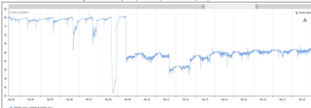
Figura 1 - Mudança de pressão após início da operação da VRP
