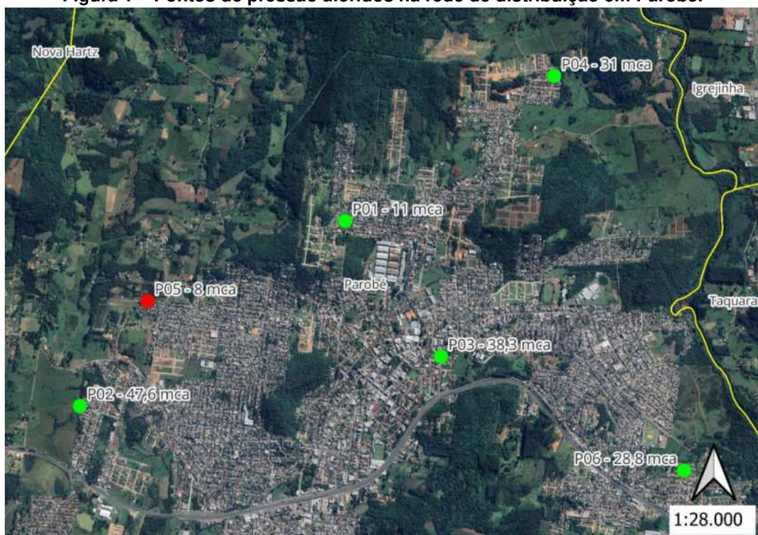
Figura 1 – Pontos de pressão aferidos na rede de distribuição em Parobé.
