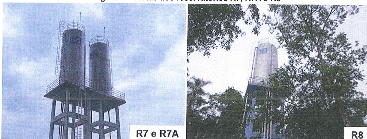
Figura 1 – Vistas dos reservatórios R7, R7A e R8
