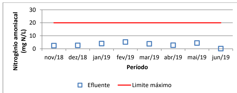
Figura 6. Monitoramento do nitrogênio amoniacal no efluente e limite máximo estabelecido na LO.
