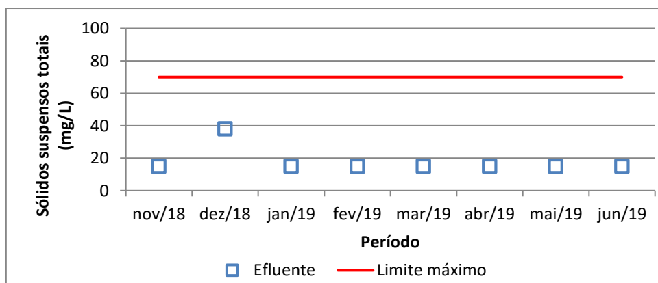
Figura 4. Monitoramento de sólidos suspensos totais no efluente e limite máximo estabelecido na LO.
