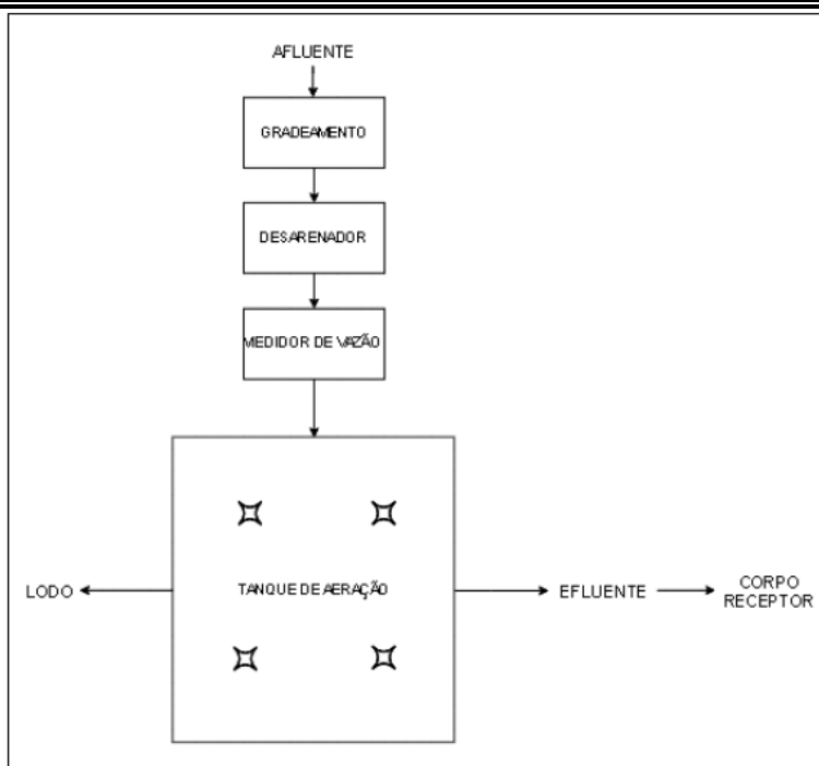
Figura 1. Esquema do sistema de tratamento da ETE Vicinal COHAB.
