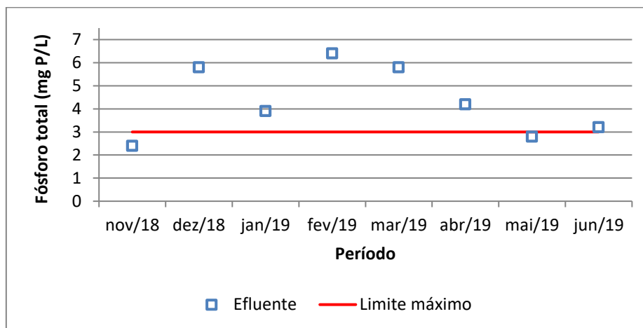
Figura 7. Monitoramento do fósforo total no efluente e limite máximo estabelecido na LO.
