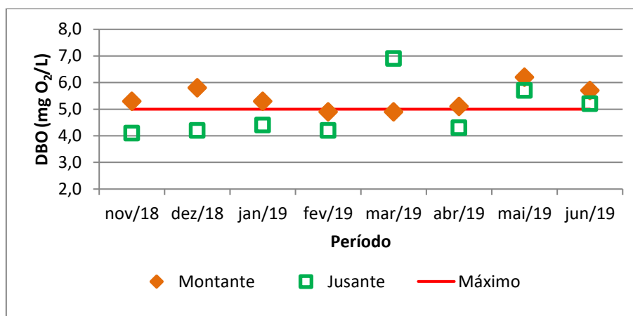
Figura 10. Monitoramento de DBO 5 no corpo receptor e limite máximo estabelecido pela CONAMA 357/2005..
