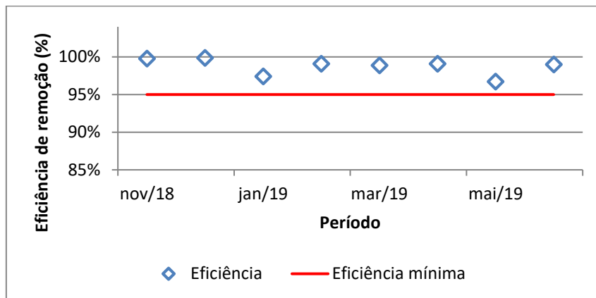
Figura 8. Monitoramento da eficiência de remoção de E. coli e eficiência mínima exigida na LO.
