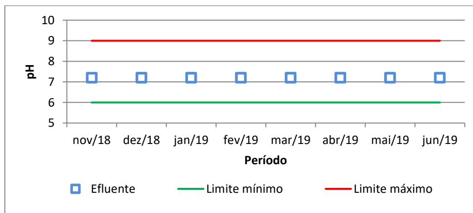
Figura 9. Monitoramento de pH no efluente e limites estabelecidos pela LO.
