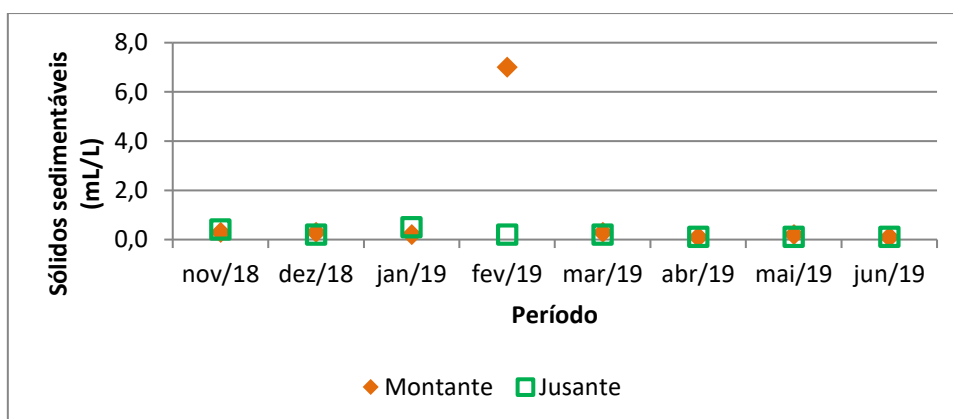
Figura 11. Monitoramento de sólidos sedimentáveis a montante e a jusante do ponto de lançamento no Arroio José Joaquim.
