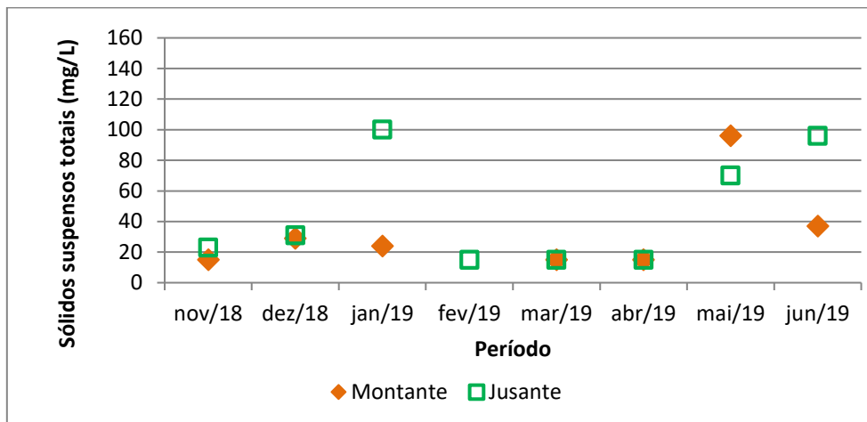
Figura 10. Monitoramento de sólidos suspensos totais a montante e a jusante do ponto de lançamento no Arroio José Joaquim.
