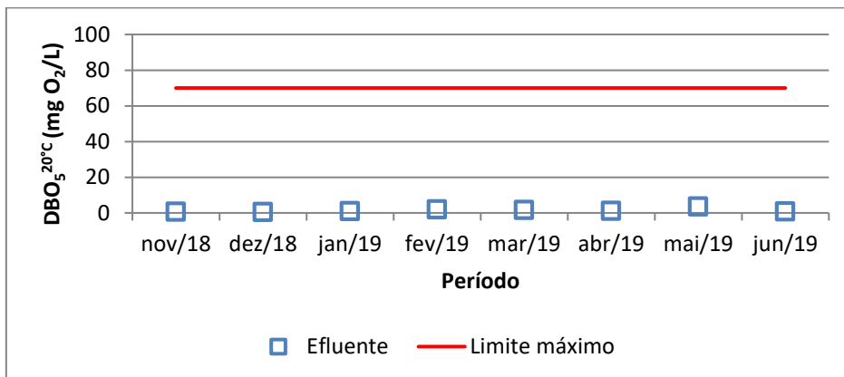
Figura 3. Monitoramento da DBO 5 no efluente e limite máximo estabelecido na LO.
