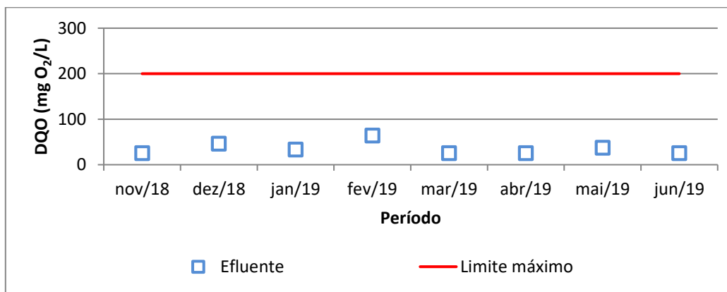
Figura 2. Monitoramento da DQO no efluente e limite máximo estabelecido na LO.
