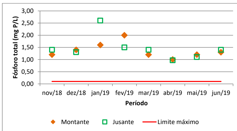
Figura 14. Monitoramento do fósforo total a montante e a jusante do lançamento no corpo receptor e o limite estabelecido na legislação.
