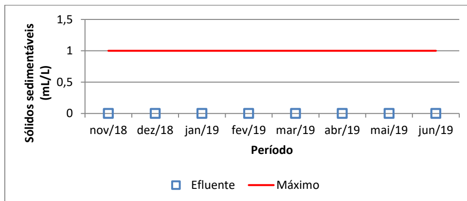
Figura 5. Monitoramento de sólidos sedimentáveis no efluente e limite máximo estabelecido pela LO.
