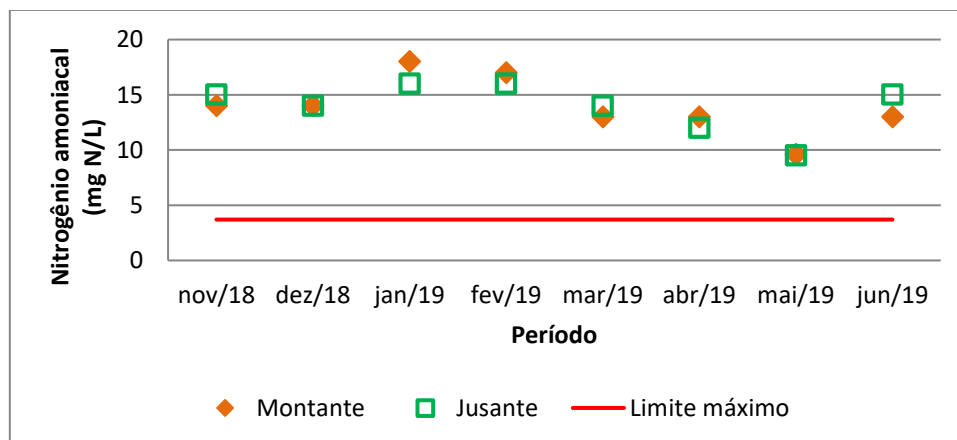
Figura 13. Monitoramento do nitrogênio amoniacal a montante e a jusante do lançamento no corpo receptor e o limite estabelecido na legislação.
