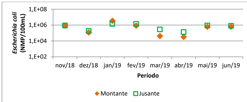
Figura 12. Monitoramento de E. coli a montante e a jusante do ponto de lançamento no Arroio José Joaquim.
