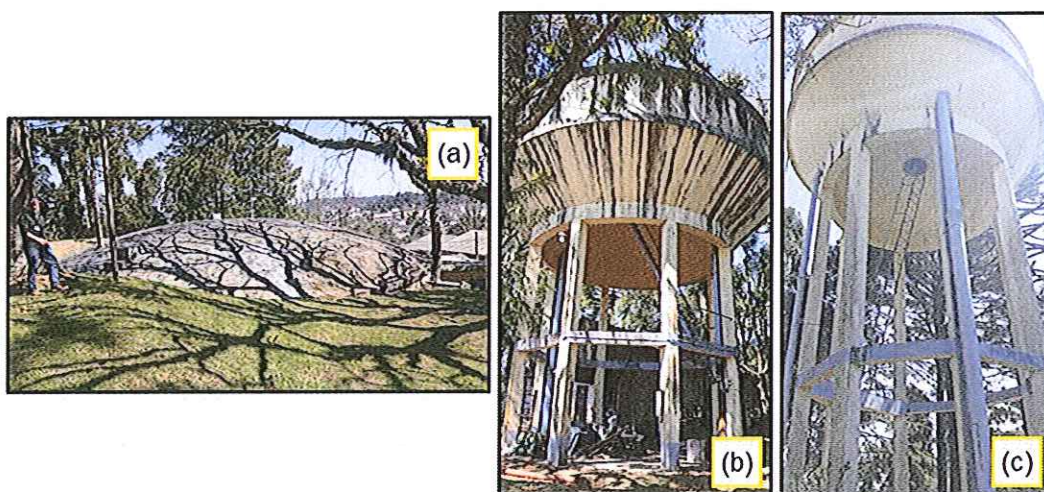
Figura 6: Reservatórios localizados junto à ETA – I, onde (a) reservatório R-03 de 1.500 m 3 ; (b) reservatório R-4 de 250 m 3 , e; (c) reservatório R-5 de 100 m 3 .
