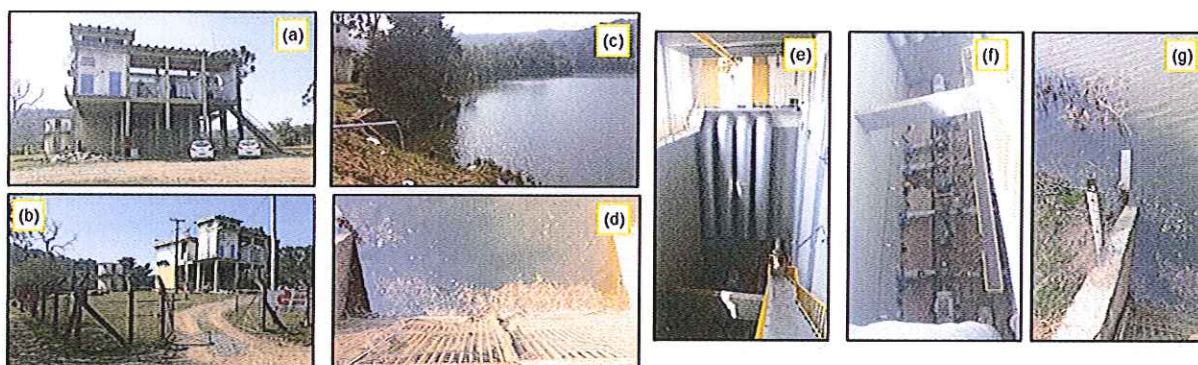
Figura 3: Registro fotográfico do local da captação, onde: (a) vista frontal da edificação; (b) portão, cercamento e estrada de acesso, (c) ponto de captação; (d) detalhe do ponto de captação com peneira e gradeamento; (e-f) casa de bombas, e; (g) marcadores de nível do manancial.
