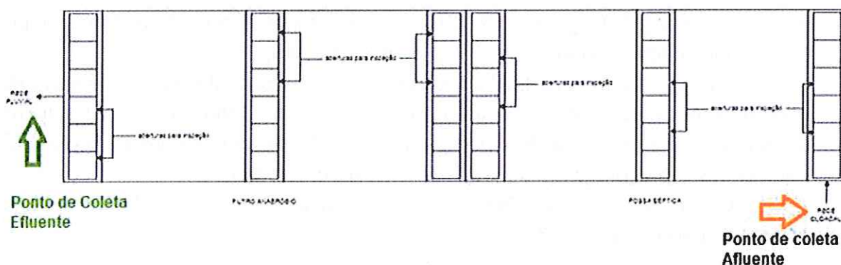
Figura 2: Diagrama esquemático do sistema da ETE Loteamento Munari e seus respectivos pontos de coleta do afluente e efluente. Fonte: CORSAN.
