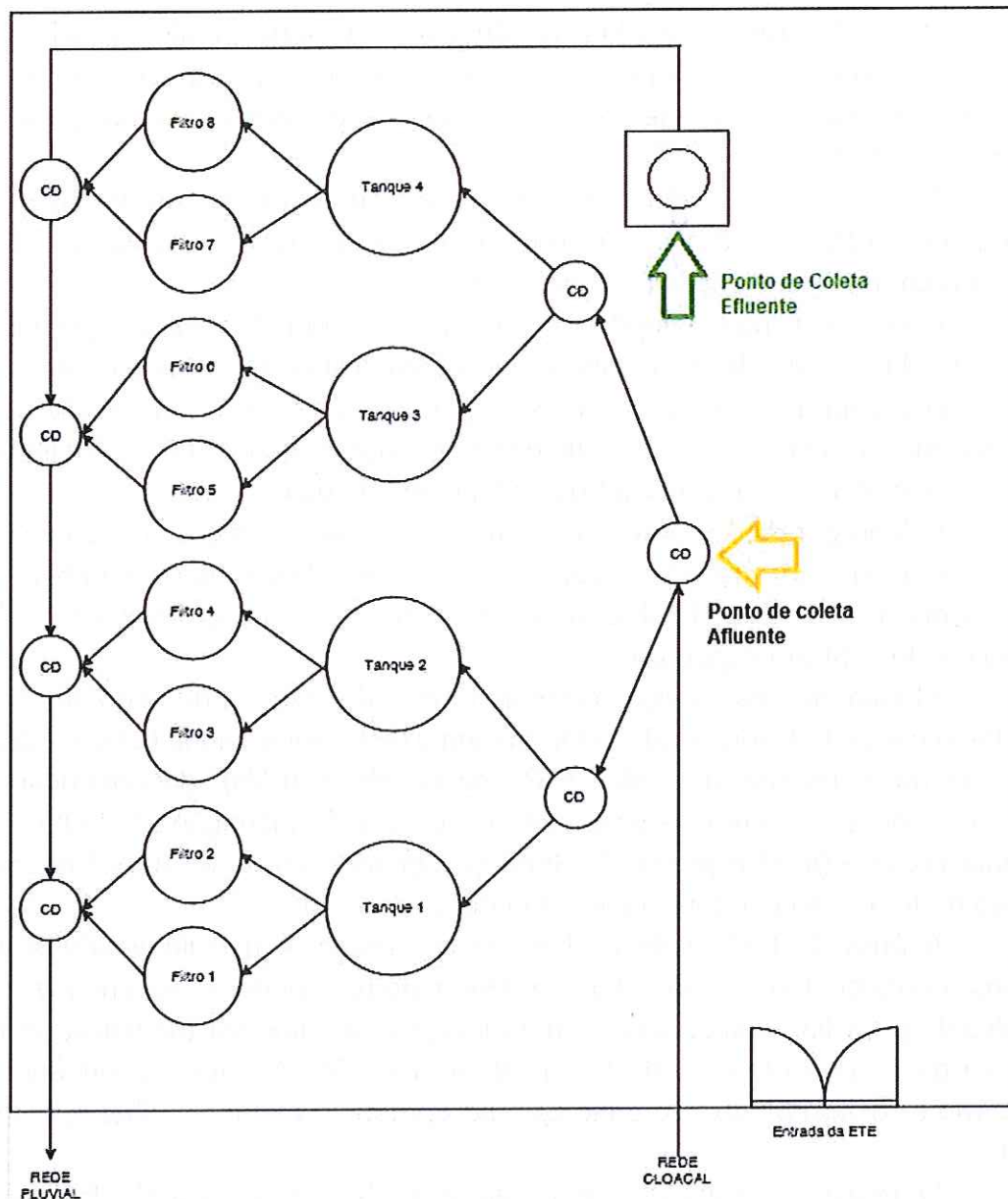
Figura 2: Diagrama esquemático do sistema da ETE Loteamento Horizonte e seus respectivos pontos de coleta do afluente e efluente. Fonte: CORSAN.
