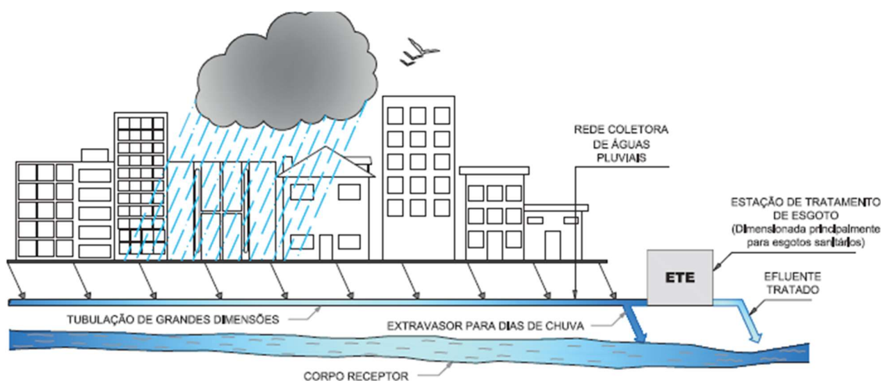
Figura 4 – Esquema ilustrativo do Sistema Unitário
