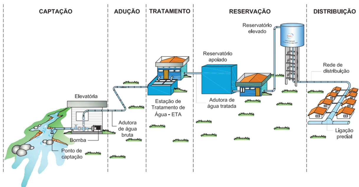
Figura 1 – Esquema ilustrativo de um Sistema de Abastecimento de Água (SAA)
