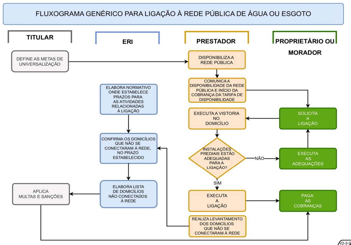
Figura 8 – Fluxograma genérico para ligação à rede pública de água ou esgoto
