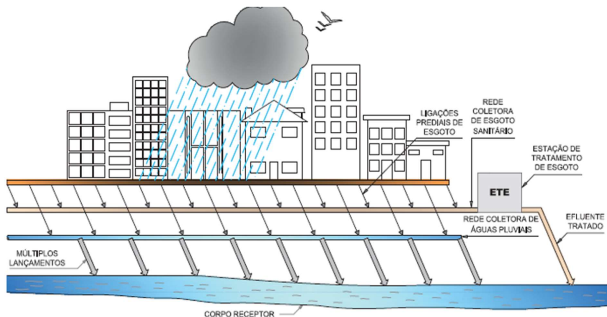
Figura 3 – Esquema ilustrativo do Sistema Separador Absoluto
